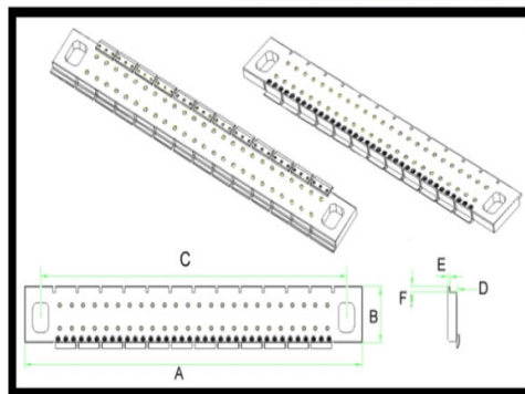
Traversa Bilaterale SU-TR-901-n-x
