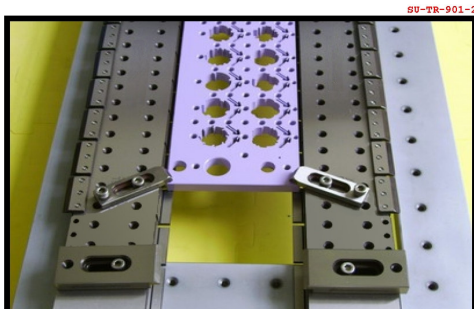
Traverse (Ruler) & Blocco "V"
